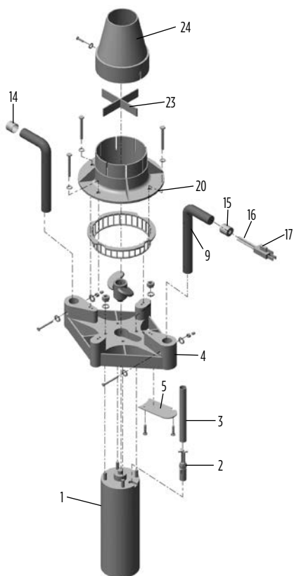
Figura 12 Vista de despiece: Montaje de la bomba de oxigenación
