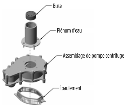
Illustration 14 Vue éclatée – Trousse de conversion de tête de pompe centrifuge
