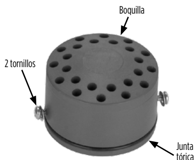
Figura 15 Montaje de boquilla para fuente decorativa (Nota: La boquilla Staccato se muestra a modo de referencia).
