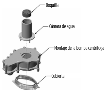
Figura 14 Vista de despiece: Juego de conversión de cabezal de bomba centrífuga
