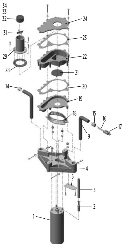
Figura 13 Vista de despiece: Montaje de la bomba centrífuga
